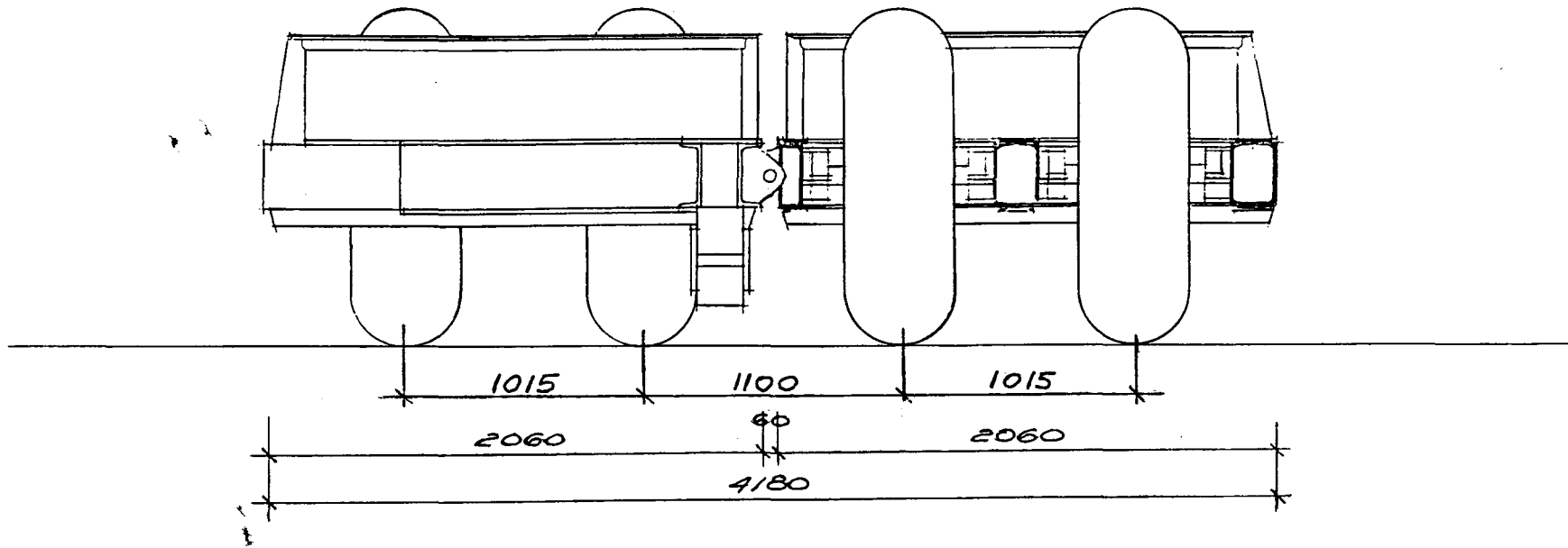
END ELEVATION
